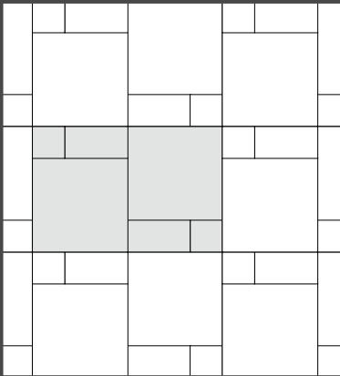
60,9x60,9=75% 20,3x40,6=16,7% 20,3x20,3=8,3% K
