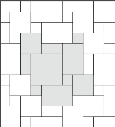
60,9x60,9=25% 40,6x60,9=33,3% 40,6x40,6=22,2% 20,3x40,6=11,1% 20,3x20,3=8,3% M
