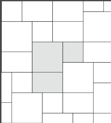
60x60=47,4% 40x60=31,6% 40x40=21,1% K1
